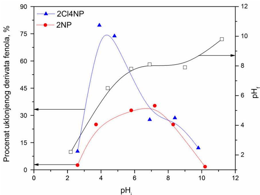
Slika 26. Uticaj pH na sorpciju 2NP i 2Cl4NP na CP-S A -deta i pH_f = f(pH_i) dijagram
