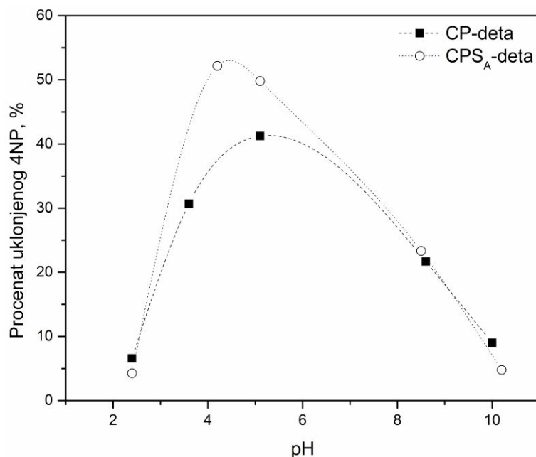
Slika 17. Uticaj pH na sorpciju 4NP na CP-deta i CP-S A -deta na 25 °C, m_{\text{sorb}} = 25 \text{ mg} , C_0 = 2 \times 10^{-4} \text{ mol dm}^{-3}
