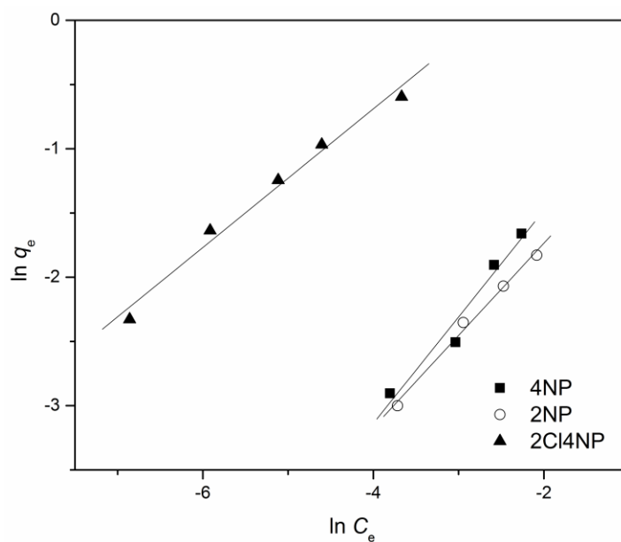
Slika 32. Freundlihovala izoterma za adsorpciju 4NP, 2NP i 2Cl4NP na CP-S A -deta
