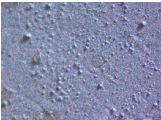
Slika 6 - Morfologija prevlaka Zn-Mn legura dobijenih taloženjem gustinom struje od 5 \text{ A dm}^{-2} iz pirofosfatnog rastvora (uvećanje 20 \times )
