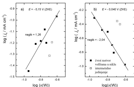
Slika 6 - a) Vrednosti katodnih gustina struja pri potencijalu -0,150 V (ZKE) u zavisnosti od molskog udela volframa u leguri; b) Vrednosti anodnih gustina struja pri potencijalu -0,040 V (ZKE) u zavisnosti od molskog udela volframa u leguri; rastvor 0,5 mol dm^{-3} H_2SO_4
