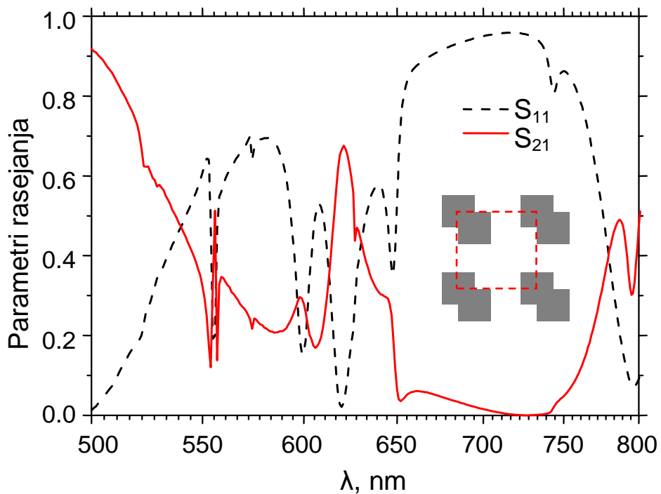
Slika 6.6.3 Koeficijent refleksije ( S_{11} ) i transmisije ( S_{21} ) jedinične superćelije za pomeraj od 50% između osnovnog i preslikanog kvadrata.
