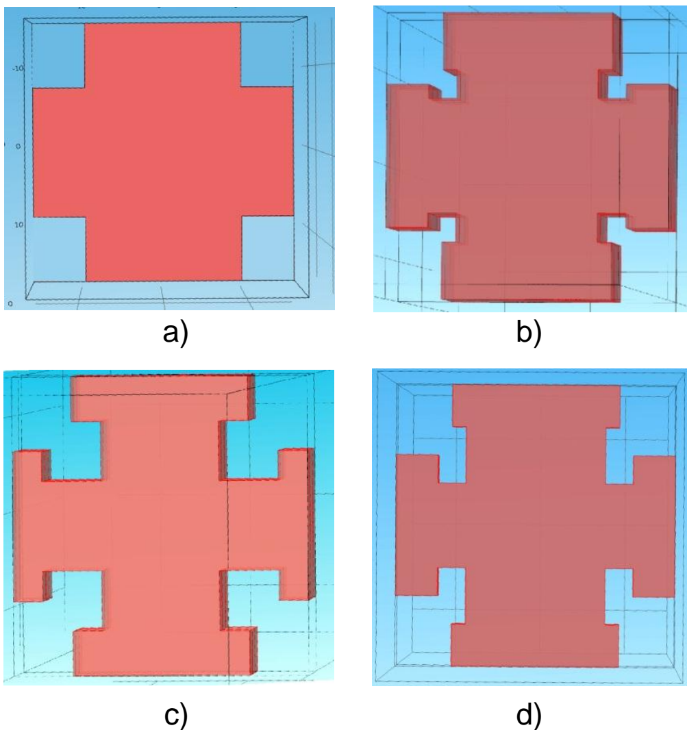
Slika 6.5.3 Prikaz jediničnih ćelija modelovanih programom COMSOL Multiphysics. a) osnovni oblik bez podotvora, b) jedinična superćelija sa dodatnim kvadratnim podotvorima dimenzija 30\text{ nm} \times 30\text{ nm} na uglovima osnovnog kvadratnog otvora, c) sa dodatnim kvadratnim podotvorima dimenzija 60\text{ nm} \times 60\text{ nm} i d) sa dodatnim pravougaonim podotvorima dimenzija 30\text{ nm} \times 60\text{ nm} .
