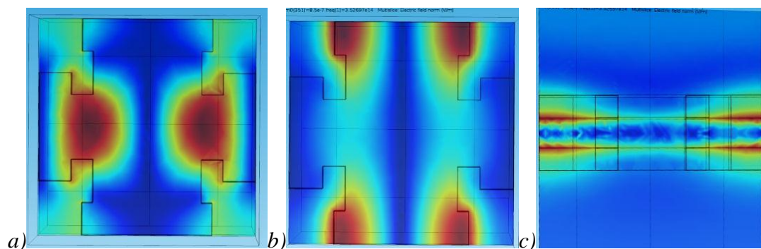
Slika 6.5.14 Prostorna raspodela električnog polja u superćeliji izračunata programom COMSOL Multiphysics. Prema spektralnoj zavisnosti prikazanoj na slici 6.5.5 i na: a) \lambda=650 nm, presek po x-y ravni na sredini strukture b) \lambda=850 nm, presek po x-y ravni i c) \lambda=850 nm, po x-z ravni.
