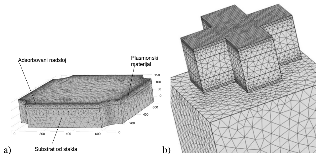
Sl. 5.2.6 a) Jedinična ćelija jednoslojnog plazmonskog mrežastog metamaterijala na staklu sa adsorbovanim monoatomskim slojem i generisanom mrežom za simulaciju u paketu COMSOL Multiphysics; b) jedinična ćelija dvostrukog mrežastog metamaterijala na podlozi i sa monoatomskim nadslojem, sa prikazanom generisanom mrežom za simulaciju u paketu COMSOL Multiphysics.
