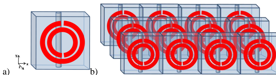
Slika 3.3.3 Evolucija stvaranja metamaterijala sa n < 0 kombinacijom dveju struktura; a) početna konfiguracija sa dvostrukim metalnim prstenovima kružnog oblika sa procepom (SRR) i žičanim medijumom ili induktivnom trakom.
