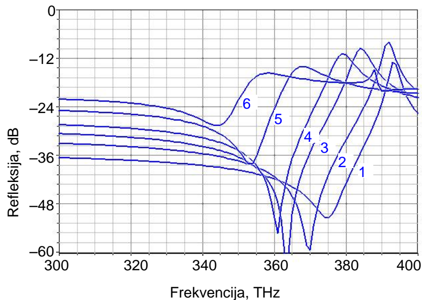
Slika 6.2.3 Uporedni dijagram koeficijenta refleksije za dvostruki mrežasti metamaterijal, debljina metala je d_m=5 nm, a debljine dielektrika: 1) 20nm, 2) 50nm, 3) 75nm, 4) 100 nm, 5) 150nm i 6) 200nm. Relativna permitivnost dielektrika je \epsilon=2 .
