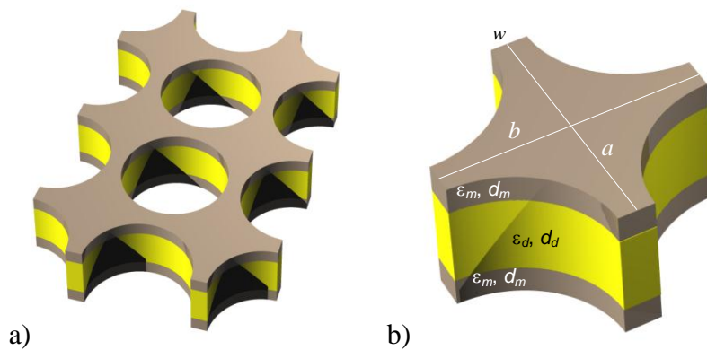
Slika 6.2.2 a) Segment dvostrukog mrežastog metamaterijala bez podloge sa kvadratnom kristalnom rešetkom; b) Jedinična ćelija modelovanog metamaterijala. Osnovni parametri strukture su naznačani na slici.
