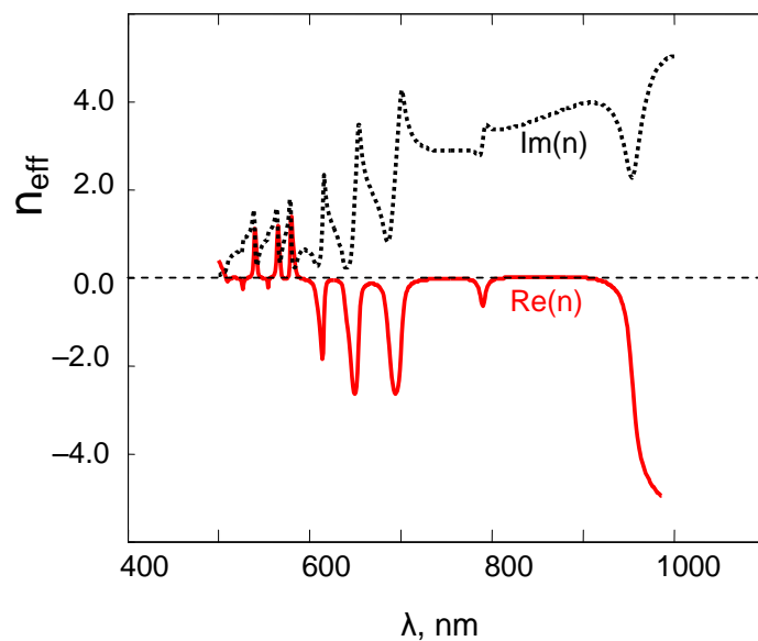
Slika 6.6.10 Efektivni indeks prelamanja dvostruke mrežaste strukture sa superćelijama sa repliciranim motivom kod koje je pomenost između preslikanih otvora 90%. Tačkastom linijom označene su imaginarne vrednosti efektivnog indeksa prelamanja, a punom linijom realne vrednosti.
