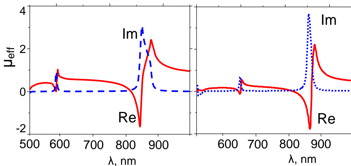
Slika 6.5.11 Izračunate vrednosti efektivne relativne magnetne permeabilnosti za osnovnu strukuru (levo) i strukturu sa podobjekom dimenzija 30\text{nm} \times 60\text{nm} (desno).
