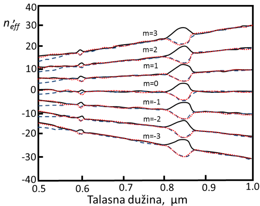
Slika 3.5.2 Prikaz izračunatih vrednosti za realnu vrednost indeksa prelamanja za m = -3 , za najnižu granu i do m=3 . Tačkaste i isprekidane grane se izračunavaju ako se poštuje pravilo da se uzima pozitivna vrednost imaginarnog dela. Puna linija je za slučaj kada se ne vodi računa o znaku.
