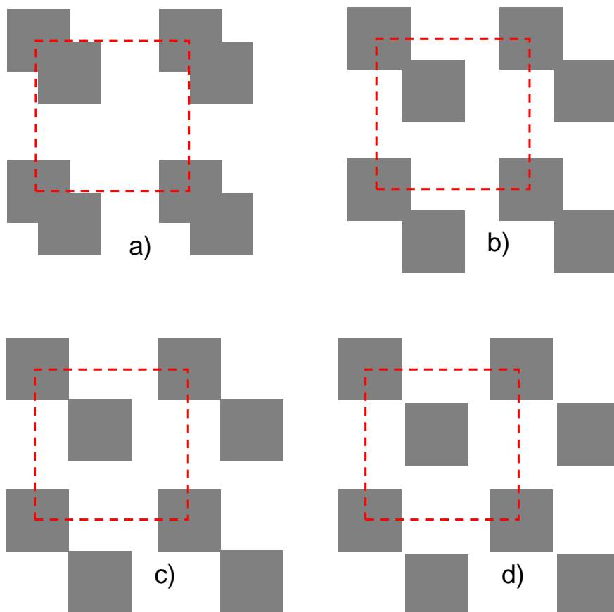
Slika 6.6.1 Četiri glavna obrasca prema kojima su formirane jedinične superćelije. a) superstruktura formirana od niza identičnih otvora pomerenih za polovinu stranice početnog otvora duž obe ose, b) pomeraj od 90% duž obe stranice, c) pomeraj od 100% duž obe stranice i d) pomeraj od 110% duž obe strane, tako da ne dolazi do preklapanja otvora. Kvadrati crtani isprekidanim linijama označavaju jediničnu ćeliju.
