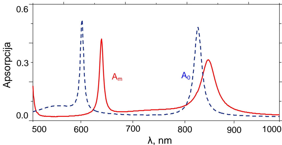
Slika 6.5.8 Koeficijent apsorpcije na neperturbovanoj osnovnoj ćeliji ( A_0 , isprekidana linija) i na superćeliji sa podotvorima 30 nm x 60 nm ( A_m , puna linija).
