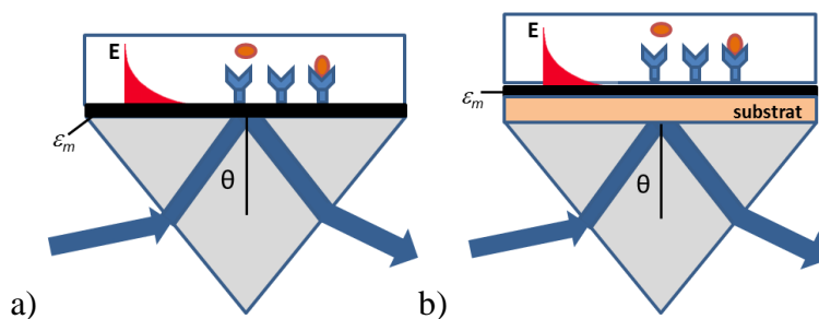
Slika 2.4.1 Šematski prikaz konfiguracija SPR senzora sa sprežnom prizmom. a) Kretschman-ova konfiguracija, b) Otto-konfiguracija
