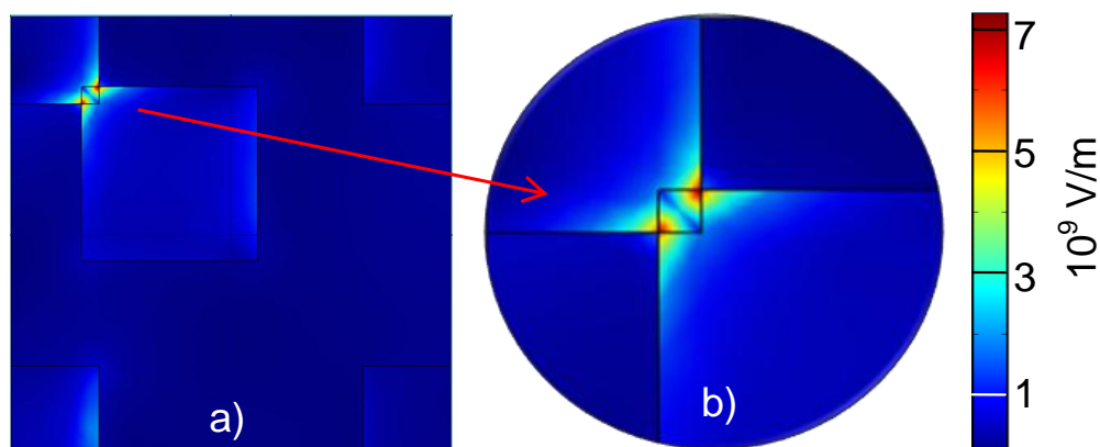
Slika 6.6.6 Profil prostorne raspodele amplitude električnog polja u superćeliji na rezonantnoj učestanosti od 638 nm; superćelija je formirana prema obrascu na slici 2b), gde je pomenost između osnovnog i preslikanog kvadrata 90%, a) cela jedinična ćelija i b) povećan deo slike sa ostrim ivicama na jediničnoj ćeliji sa dubokom podtalasnom lokalizacijom intenziteta električnog polja. Prema spektralnoj raspodeli na slici 6.6.4.
