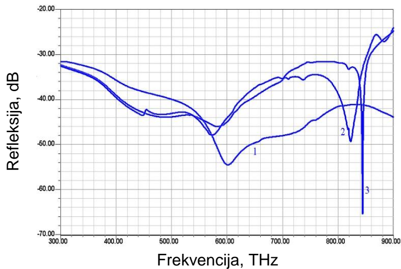
Slika 6.2.7 Uporedni dijagram za dvostruki slobodnostojeći dvostruki mrežasti metamaterijal, metal je srebro (5 nm), dielektrik kvarcno staklo (10 nm, \epsilon = 3.78 ), za različite dielektrične permitivnosti sredine u kojoj se nalazi metamaterijalna struktura: 1) \epsilon = 1 , 2) \epsilon = 1.3 , 3) \epsilon = 1.35
