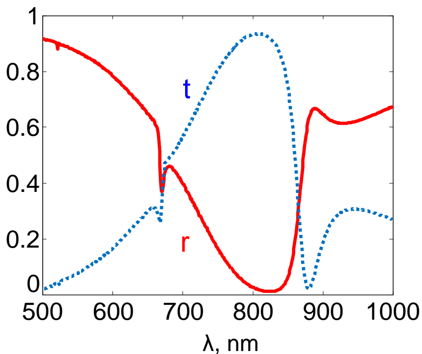
Slika 6.5.7 Transmisija i refleksija superćelije sa podbolicima na uglovima osnovnoglika u obliku kvadrata dimenzija 60 \text{ nm} \times 60 \text{ nm} .
