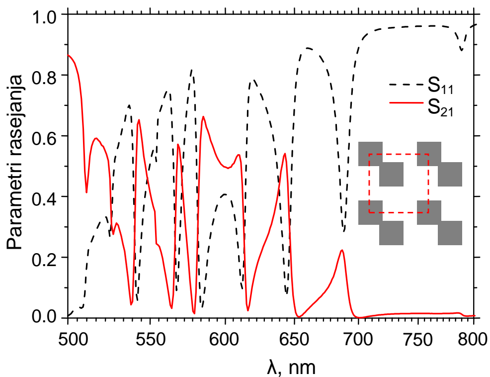
Slika 6.6.4 Koeficijent refleksije ( S_{11} ) i transmisije ( S_{21} ) jedinične superćelije za pomeraj od 90% između osnovnog i preslikanog kvadrata.
