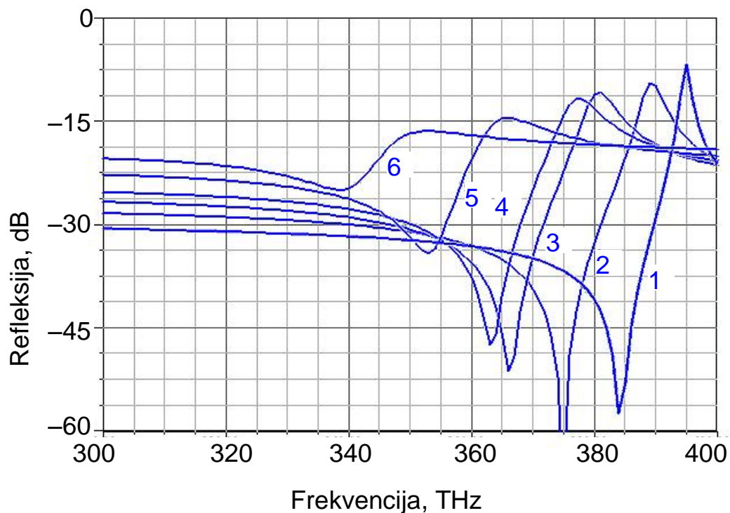
Slika 6.2.4 Uporedni dijagram koeficijenata refleksije za dvostruku mrežastu strukturu PEC-dielektrik-PEC, debljina metala je d_m=10 nm i za različite debljine dielektrika, 1) 20 nm, 2) 50 nm, 3) 75 nm, 4) 100 nm, 5) 150 nm and 6) 200 nm. Relativna permitivnost dielektrika je \epsilon=2 .
