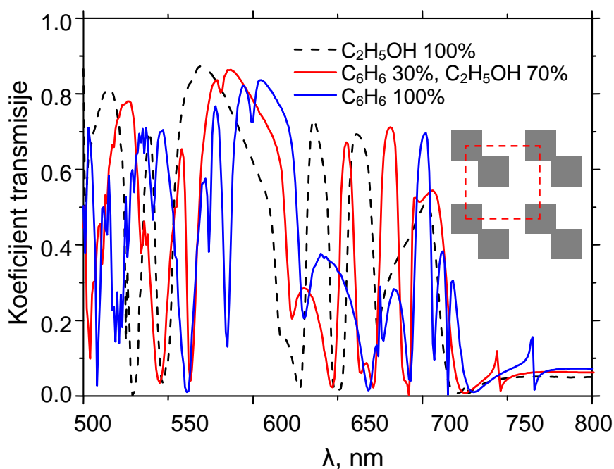
Slika 6.6.11 Parametri transmisije ( S_{21} ) superćelije formirane prema obrascu ilustrovanom na slici 2 b), gde je pomenost 90% između osnovnog i preslikanog kvadrata za tri različita medijuma, čist etanol (isprekidana linija), smešu 30% benzena i 70% etanola (crvena puna linija), i čist benzen (plava puna linija).
