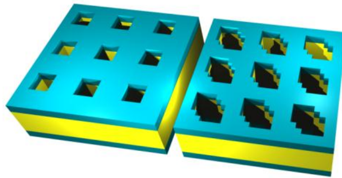
Slika 3.3.10 Dvostruka mrežasta struktura (metal-dielektrik-metal) a) otvori su kvadratni, razmešteni u kvadratnoj rešetki; b) superćelijadobijena superpozicijom tri identična kvadrata [Tanasković, 2014,2]
