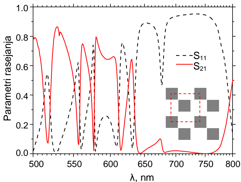
Slika 6.6.8 Spektralna refleksija ( S_{11} ) i transmisija ( S_{21} ) jedinične superćelije kada je pomeraj 110% između osnovnog i preslikanog kvadrata (nema preklapanja otvora).
