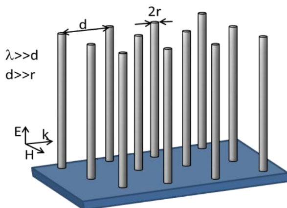
Slika 3.3. Ilustracija 2D žičanih mrežastih struktura, čija permitivnost može da bude negativna ili bliska nuli.
