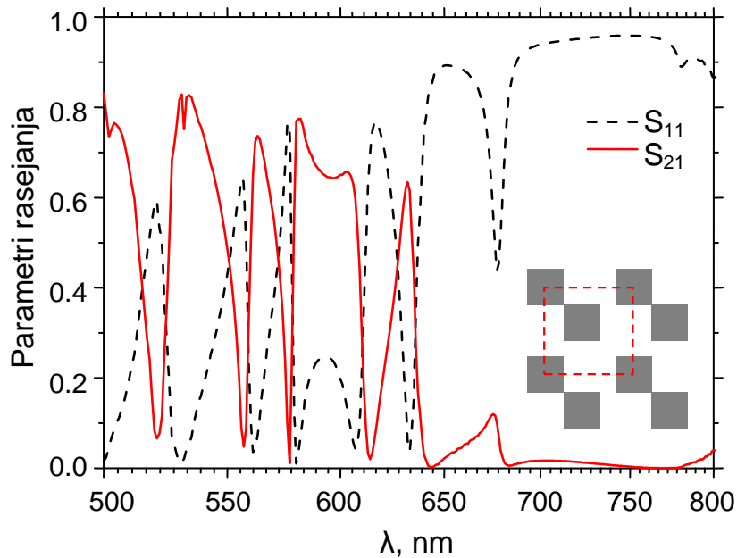
Slika 6.6.7 Spektralna refleksija ( S_{11} ) i transmisija ( S_{21} ) jediničnesuperćelije za slučaj kada je pomeraj 100% između osnovnog i preslikanog kvadrata.
