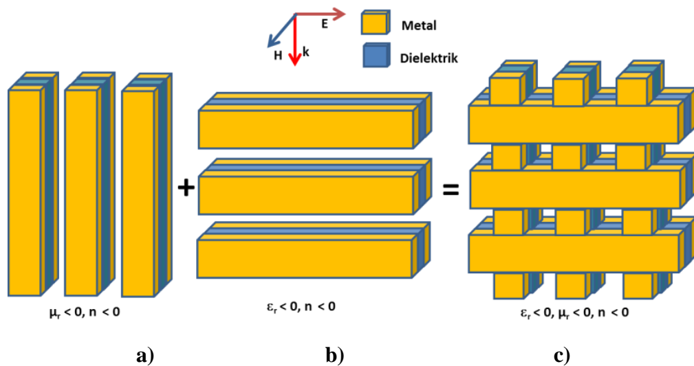
Slika 3.3.6 Evolucija stvaranja metamaterijala negativnog indeksa prelamanja kombinacijom dveju struktura; a) trake TM magnetnog metamaterijala (rezonantna struktura); b) trake (TE) električnog metamaterijala (nerezonantna struktura) i c) struktura u vidu ribarske mreže nastala integracijom prethodne dve strukture.
