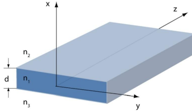
Slika 2.3.1 Ilustracija talasovoda indeksa prelamanja n_1 okruženog sredinama n_2 i n_3 . Ukoliko je n_2=n_3 reč je o simetričnom talasovodu. Širina sloja je d i ograničena je po x pravcu. Po y pravcu talasovod smatramo približno beskonačnim, a talas se prostire u pravcu z ose.
