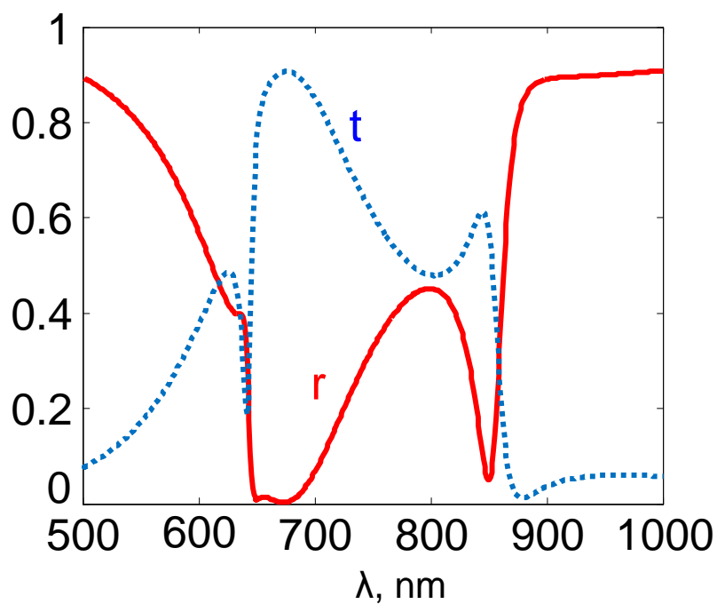
Slika 6.5.6 Transmisija i refleksija superćelije sa podobjektima na uglovima osnovnoglika u obliku kvadrata dimenzija 30 \text{ nm} \times 30 \text{ nm} .
