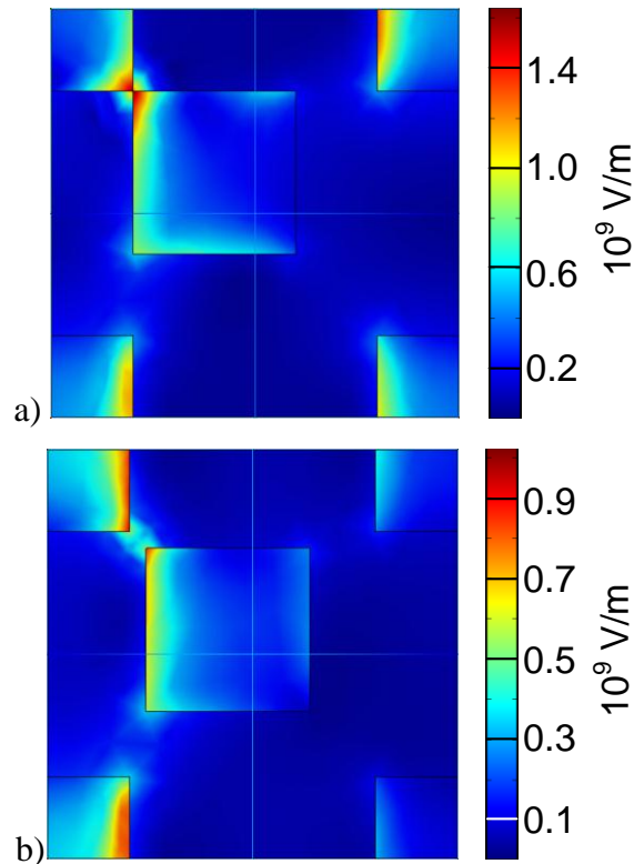
Slika 6.6.9 Profil prostorne raspodele amplitude električnog polja u superćeliji na rezonantnoj učestanosti a) od 580 nm (prema spektralnoj raspodeli na slici 6.6.7); superćelija je formirana prema likusa sl. 2b), gde je pomerenost 100% između osnovnog i preslikanog kvadrata, b) od 578 nm (prema spektralnoj raspodeli na slici 6.6.8); superćelija je formirana prema liku na slici 2b), gde je pomeraj između osnovnog i preslikanog kvadrata 110%.
