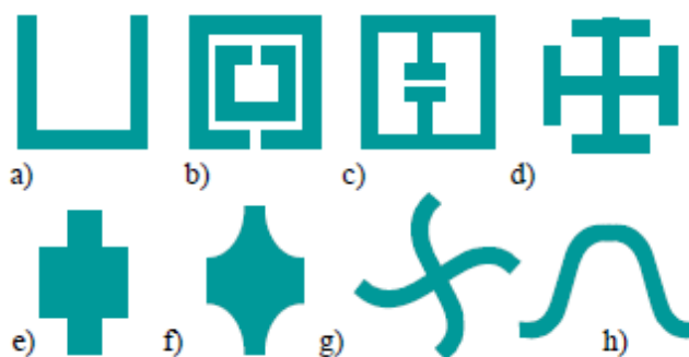
Slika 3.3.4 Primeri kontura sa metalnim slojevima za formiranje 2D metamaterijala. Od a) do d) su konstrukcije rezonantnih prstenova za magnetne metamaterijale, a u drugom redu od e) do f) su mrežasti oblici [Jakšić, 2010, 2].
