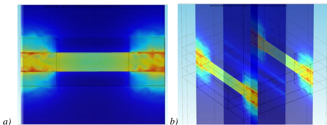
Slika 6.4.8 Poređenje profila amplitude E_x električnog polja na osnovu COMSOL Multiphysics modela za slučaj strukture sa ITO, \lambda=800\text{ nm} ; a) presek po x-y ravni na ivicama otvora; b) pogled iskosa na presek po x-z ravni na ivicama otvora.
