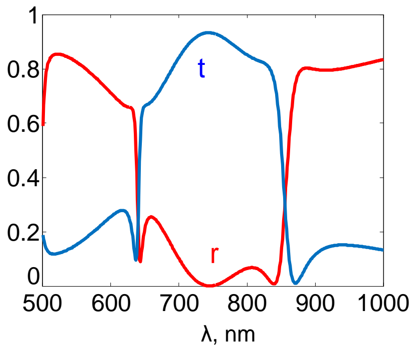
Slika 6.5.5 Transmisija i refleksija jedinične superćelije sa podobjektima na uglovima osnovnog lika u obliku pravougaonika dimenzija 30 \text{ nm} \times 60 \text{ nm} .
