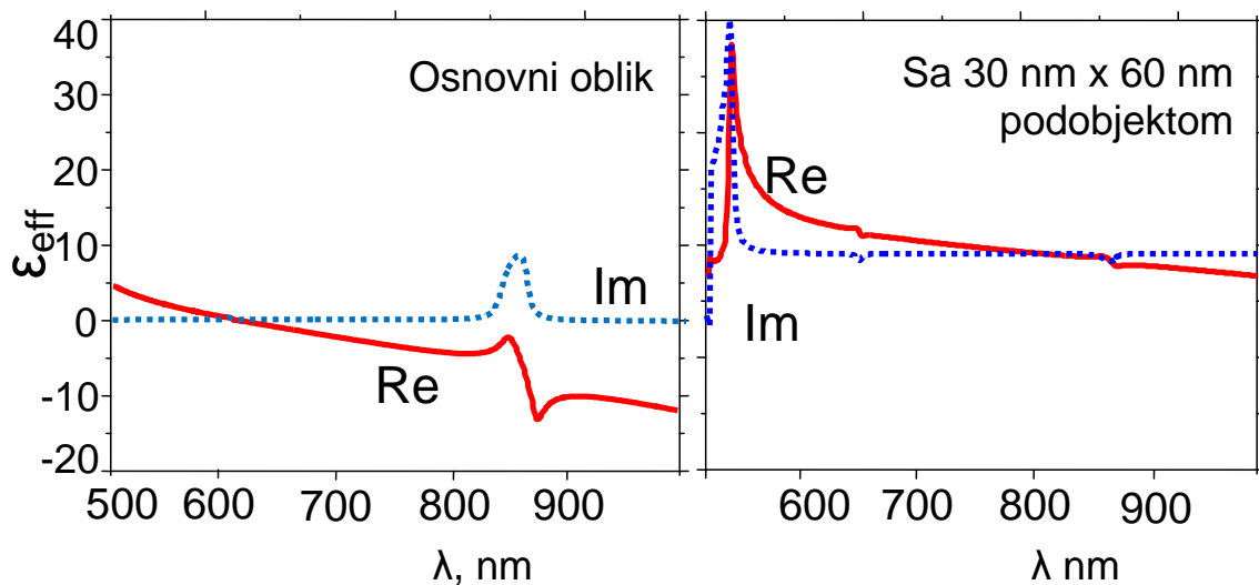
Slika 6.5.10 Izračunate vrednosti efektivne relativne dielektrične permitivnosti za osnovnu strukturu (levo) i strukturu sa podobjektom dimenzija 30 nm × 60 nm (desno).
