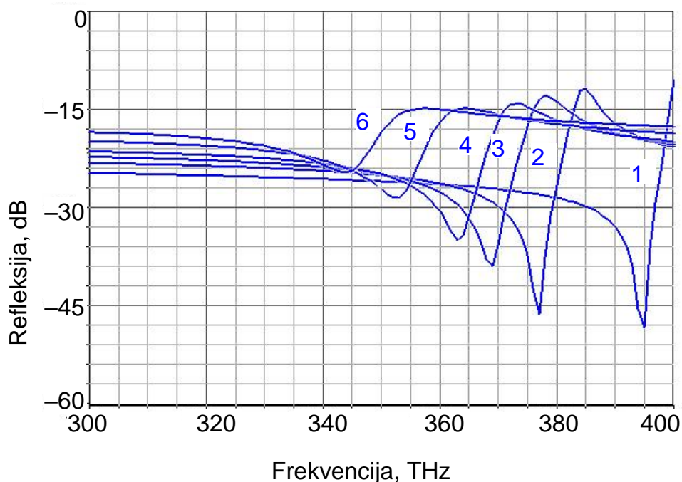
Slika 6.2.5 Uporedni dijagram za koeficijent refleksije za dvostruki mrežasti metamaterijal, debljina metala je d_m=20 nm, za različite debljine dielektrika, 1) 20 nm, 2) 50 nm, 3) 75 nm, 4) 100 nm, 5) 150 nm i 6) 200 nm. Relativna permitivnost dielektrika je \epsilon=2 .
