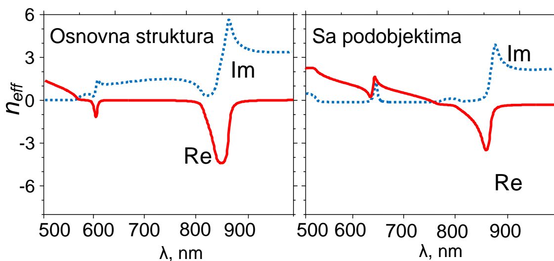
Slika 6.5.12 Izračunate vrednosti efektivnog indeksa prelamanja za osnovnu strukuru (levo) i strukturu sa podobjekom dimenzija 30\text{nm} \times 60\text{nm} (desno).
