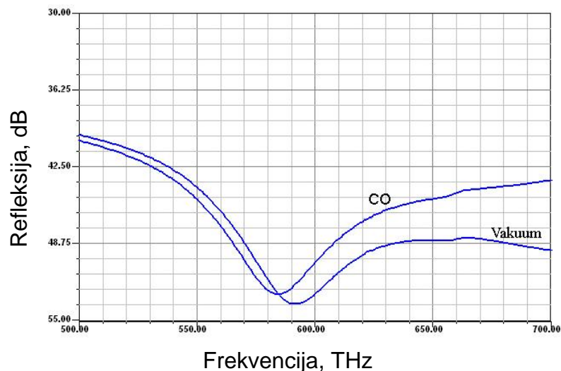
Slika 6.2.8 Uporedni dijagram za slobodnostojeći dvostruki metamaterijal, metal je srebro (5 nm), dielektrik kvarcno staklo (10 nm, \epsilon_r = 3.78 ) za dielektrične sredine: 1) \epsilon_r = 1 (vazduh), 2) \epsilon_r = 1.00634 (ugljen monoksid na 25°C).
