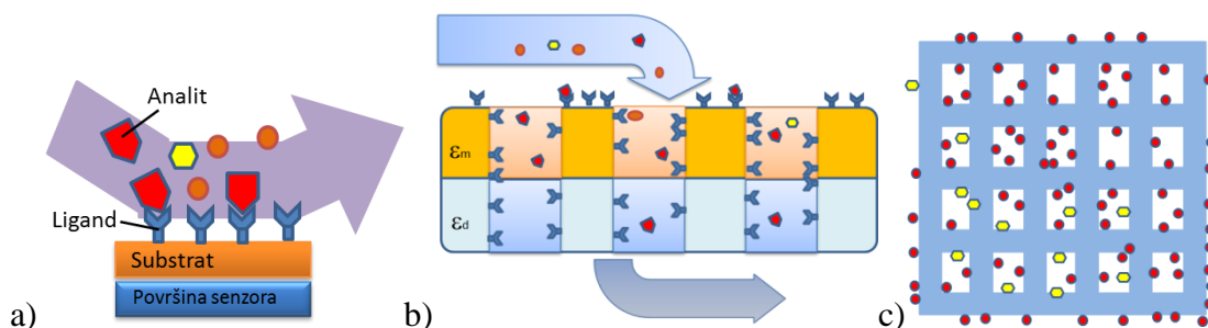
Slika.4.3.1 Ilustracija različitih načina izlaganja HBB plazmanskog senzora agensu. a) konvencionalni SPR senzor sa prizmom, b) senzor na bazi mikrofluidike u kome se koristi protok fluida sa HBB agensom kroz mrežastu metamaterijalnu strukturu i c) zapreminska adsorpcija u metamaterijalnoj strukturi.
