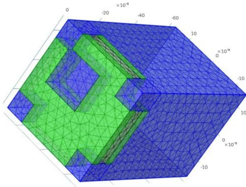
Slika 6.6.2 Jedinična superćelija sa podelom na konačne elemente kada je pomeraj od 90%, duž obe stranice, kao što je prikazano na slici 6.6.1 b).
