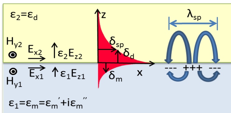
Sl. 2.3.4 Ilustracija nastajanja evanescentnog polja na međupovršini između dve sredine različitih indeksa prelamanja.
