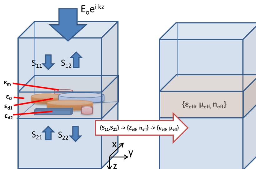
Slika 3.4.1 Ilustracija metode homogenizacije kojom se interakcija elektromagnetnog talasa i kompozitnog sistema sa elementima podtalasnih dimenzija može opisati efektivnim vrednostima optičkih parametara.
