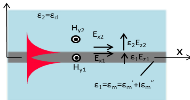
Sl. 2.3.6 Ilustracija nastajanja SPP dalekog dometa kada je tanka metalna ploča okružena dielektrikom
