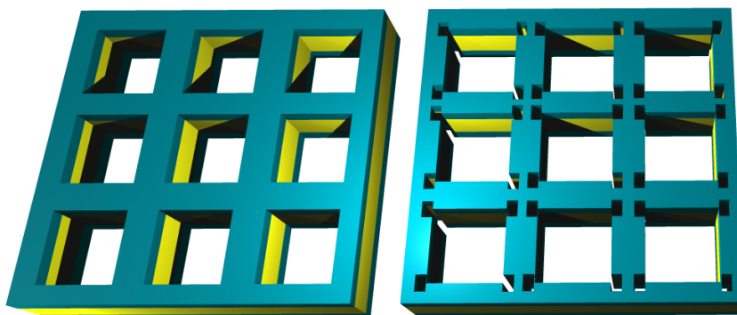
Slika 3.3.8 Prikaz uporednih ilustracija mrežaste strukture a) sa kvadratnim otvorima bez podotvora i b) superstruktura koju čine kvadratni otvori sa kvadratnim podotvorima [Tanasković, 2014,1].
