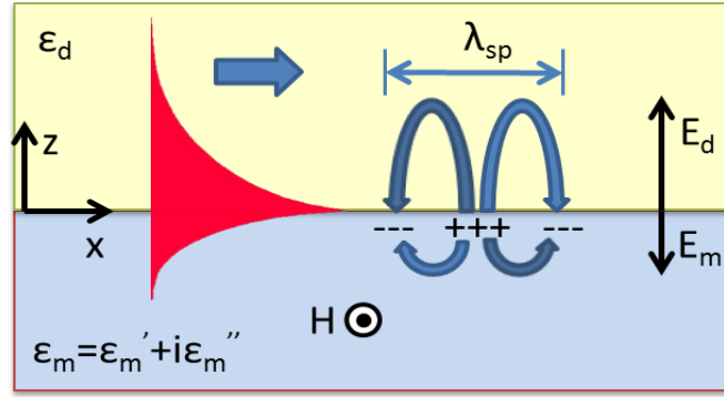
Slika 2.3.2 Šematski prikazana međupovršina metal-dielektrik sa koordinatnim sistemom i ilustracijama komponentata elektromagnetnog polja.
