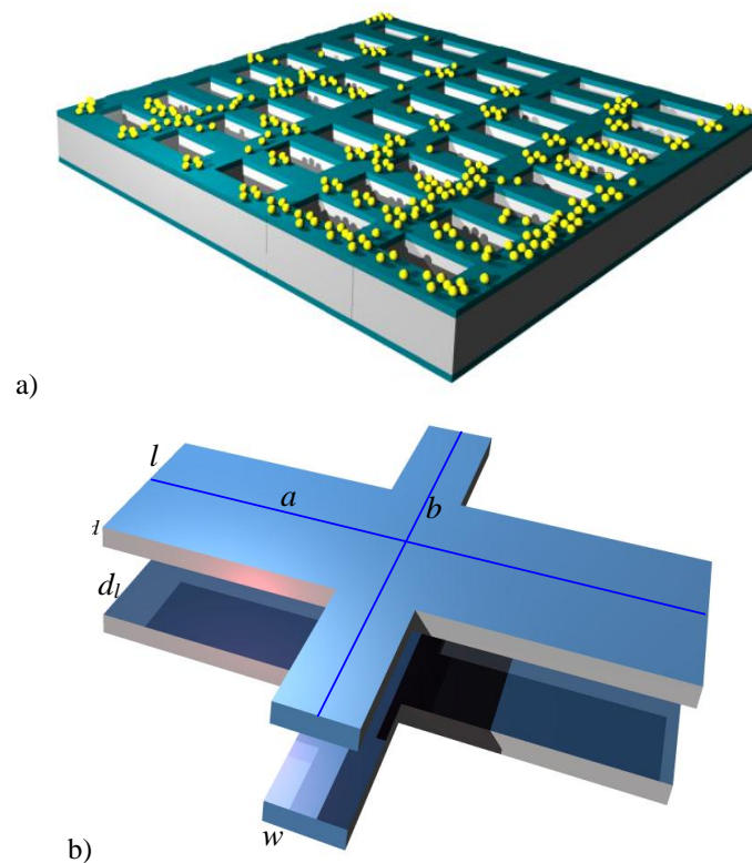
Slika 6.1.2 Geometrija jedinične ćelije dvostruke mrežaste strukture sa pravougaonim otvorima, a) mrežasta struktura sa adsorbovanim agensom simbolički prikazanim kuglicama; b) jedinična ćelija sa pravougaonim otvorima.
