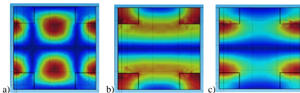
Slika 6.4.6 Poređenje profila amplitude E_x električnog polja na osnovu COMSOL Multiphysics modela za slučaj strukture sa zlatom; a) \lambda=600 nm, presek po x - y ravni na sredini strukture b) \lambda=750 nm, presek po x - y ravni i c) \lambda=900 nm, po x - y ravni.
