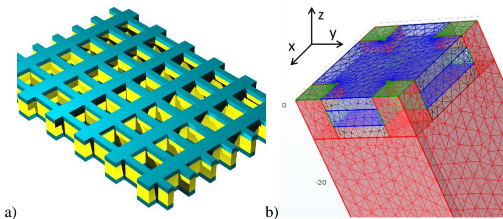
Slika 6.4.1 a) Geometrija dvostruke mrežaste strukture sa pravougaonim otvorima. b) Prikaz jedinične ćelije.
