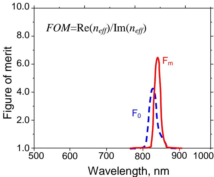
Slika 6.5.13 Izračunate vrednosti za meru kvaliteta FOM za osnovnu strukturu (isprekidana linija, označena sa 0) i strukturu sa podobjektima 30 \text{ nm} \times 60 \text{ nm} (puna linija, označena sa m).
