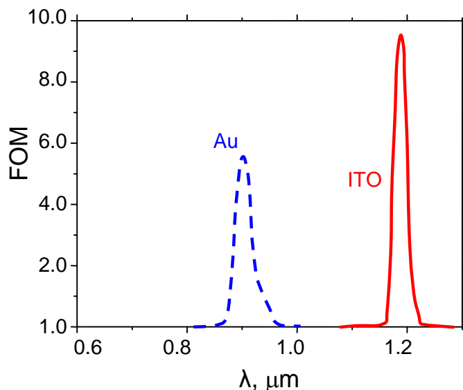
Slika 6.4. 5 Poređenje izračunatih zavisnosti mere kvaliteta FOM u slučaju strukture sa zlatom (isprekidana linija) i strukture sa ITO (puna linija)
