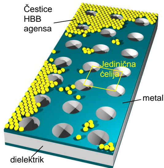
Slika 6.2.1 Generalizovana ilustracija plazmonskog senzora na bazi mrežastog metamaterijala formiranog na slobodnostojećoj nanomembrani. Kuglice simbolički predstavljaju adsorbovani HBB agens.
