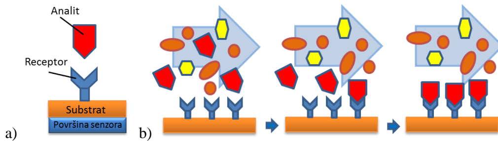
Slika 4.4.1 Šematska reprezentacija rada HBB senzora sa receptorom; a) ciljno vezivanje agensa za receptor; b) postupak detekcije u fazama, sa leve na desnu stranu, početni kontakt sa agensom, proces adsorpcije i raspoznavanja i na kraju hvatanje i povezivanje agensa za odgovarajući receptor.
